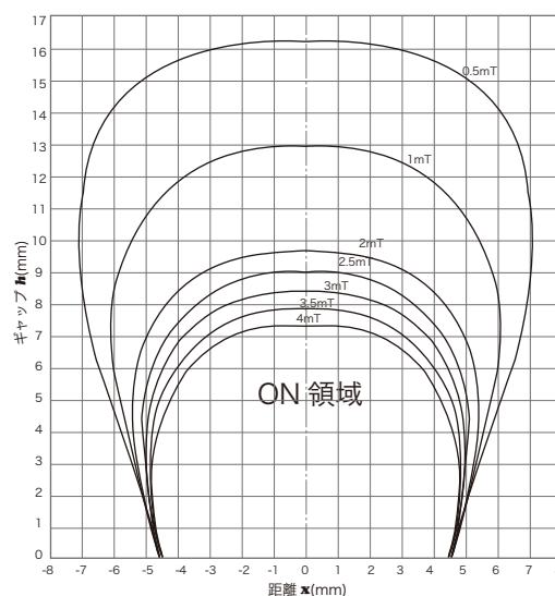
磁気特性
