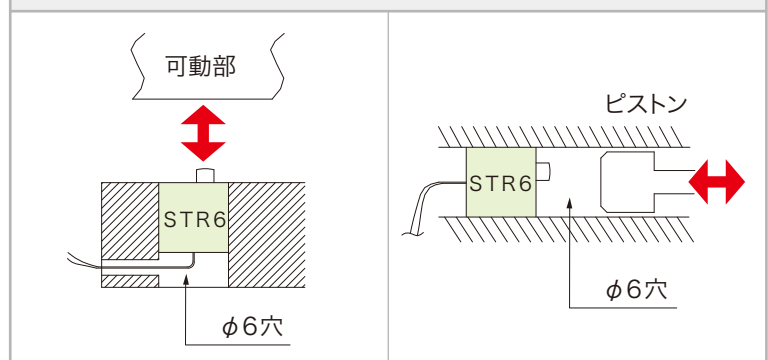
使用例 φ6のドリル穴に軽圧入で所定位置に固定
