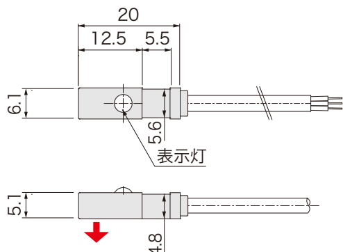
外形図
