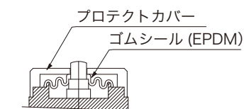
軸部のシール構造
