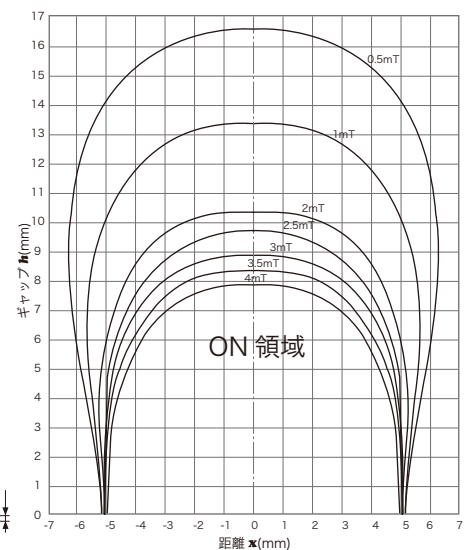
磁気特性
