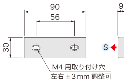
■ 外形図
