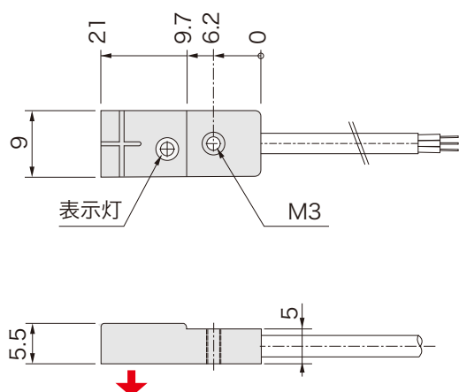
外形図
