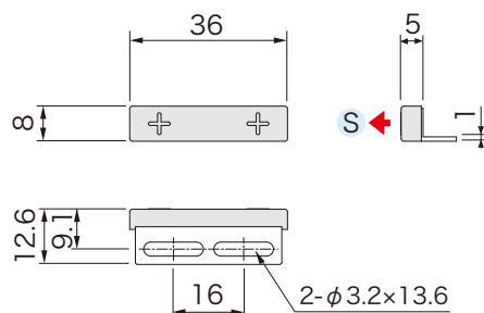
外形図
