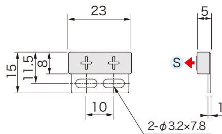
外形図
