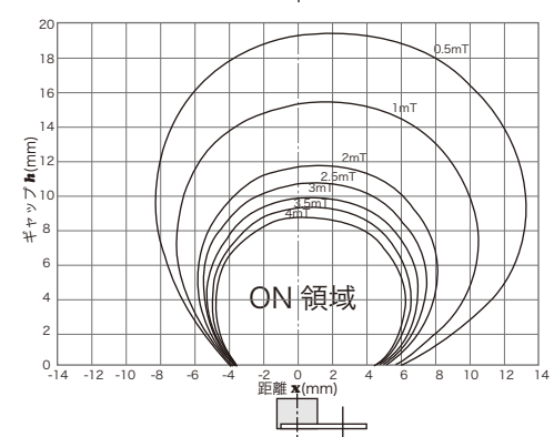
■ 磁気特性
