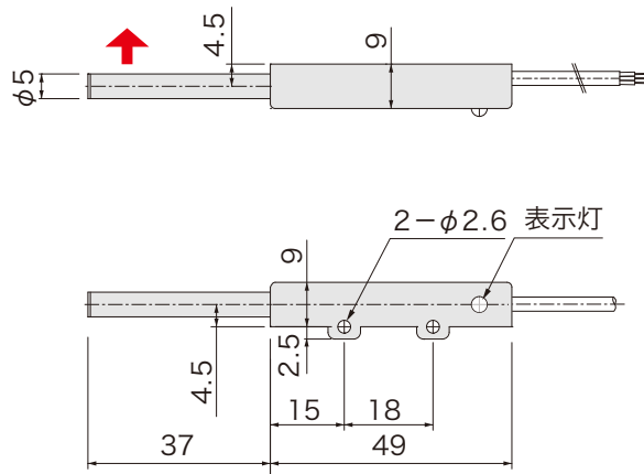
外形図
