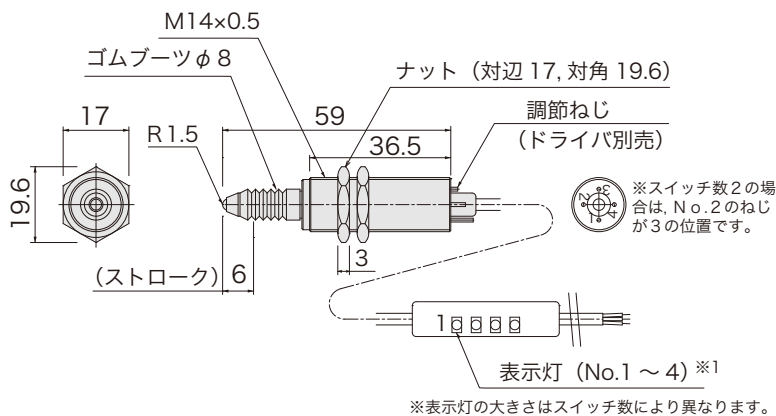
■ 外形図
