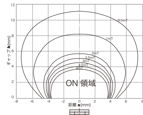
■ 磁気特性
