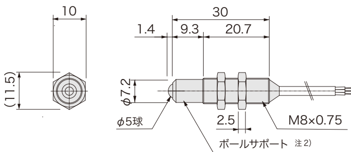
外形図
