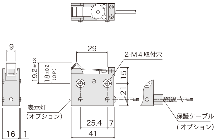
外形図
