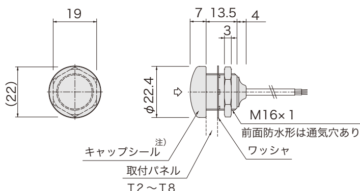
外形図
