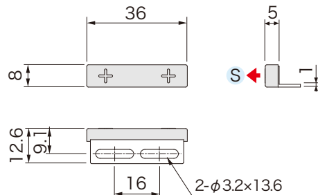
外形図
