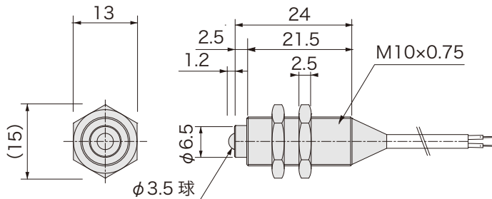
外形図
