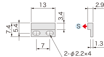
■ 外形図
