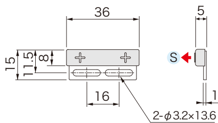
外形図
