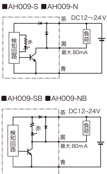
回路図
