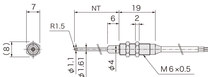
外形図
