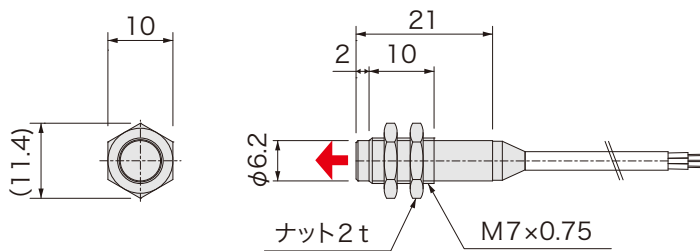
外形図
