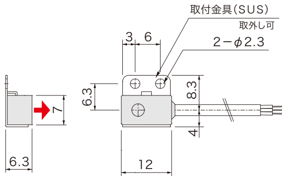
外形図
