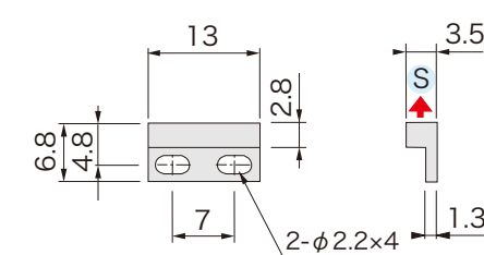
■ 外形図
