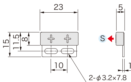
外形図
