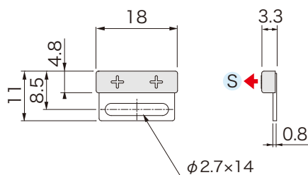
外形図
