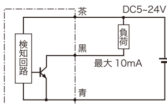
回路図
