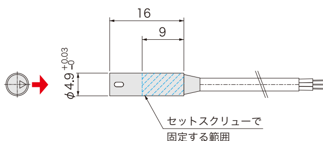
外形図
