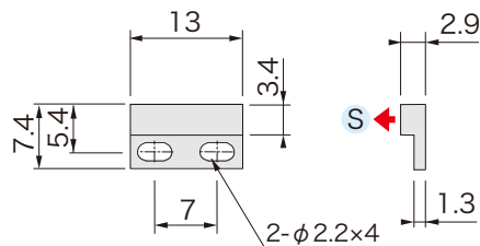
外形図
