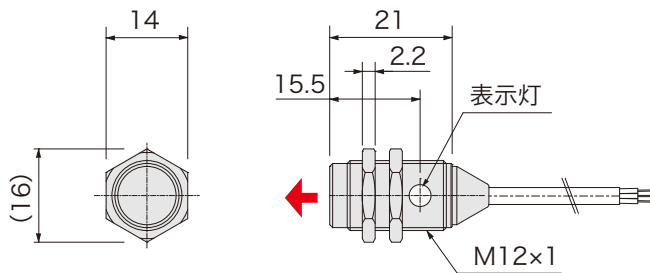
外形図
