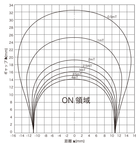
磁気特性
