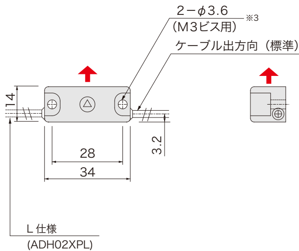
外形図
