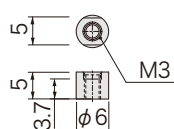
[ナット]
