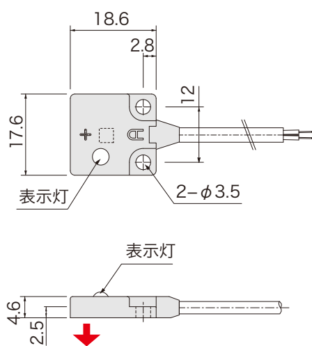
外形図
