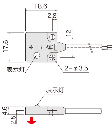
外形図
