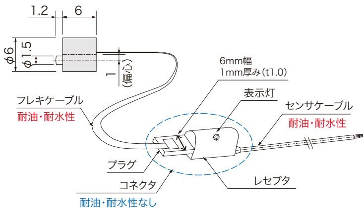
外形図
