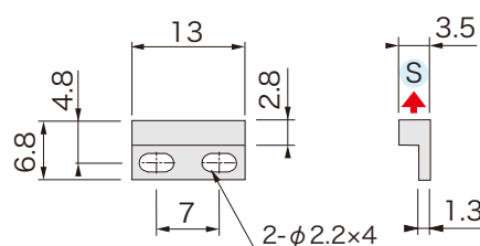
外形図
