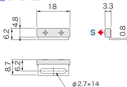
外形図
