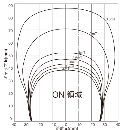
■ 磁気特性
