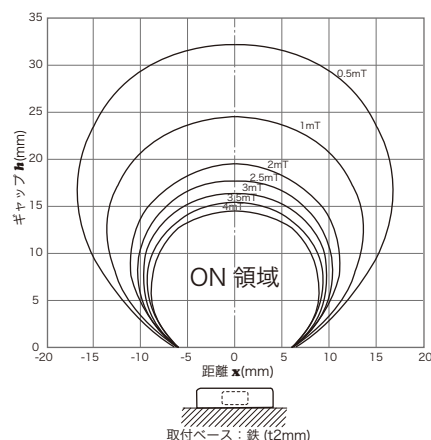
■ 磁気特性
