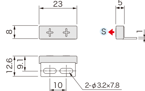
外形図
