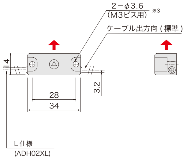
外形図
