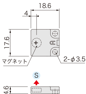
■ 外形図
