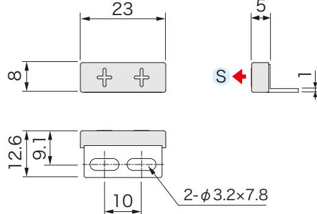
外形図
