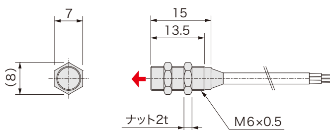
外形図
