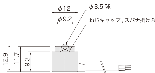
外形図
