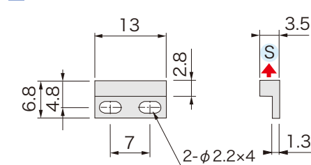
■ 外形図
