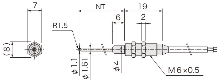
外形図
