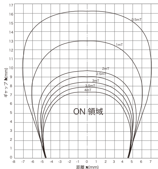
磁気特性
