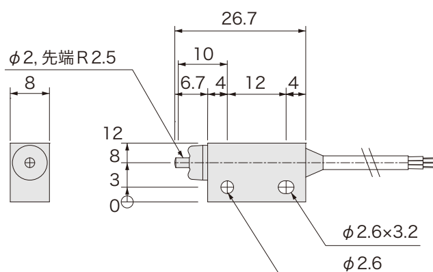
外形図
