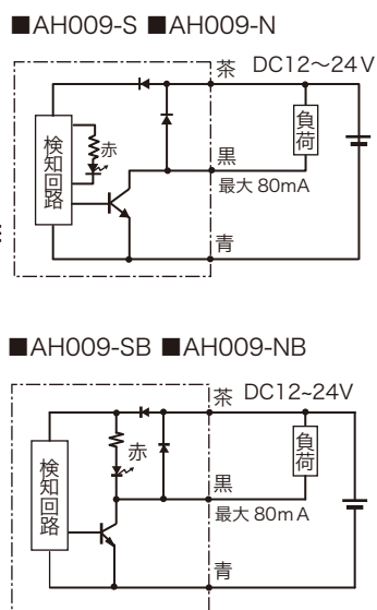
回路図
