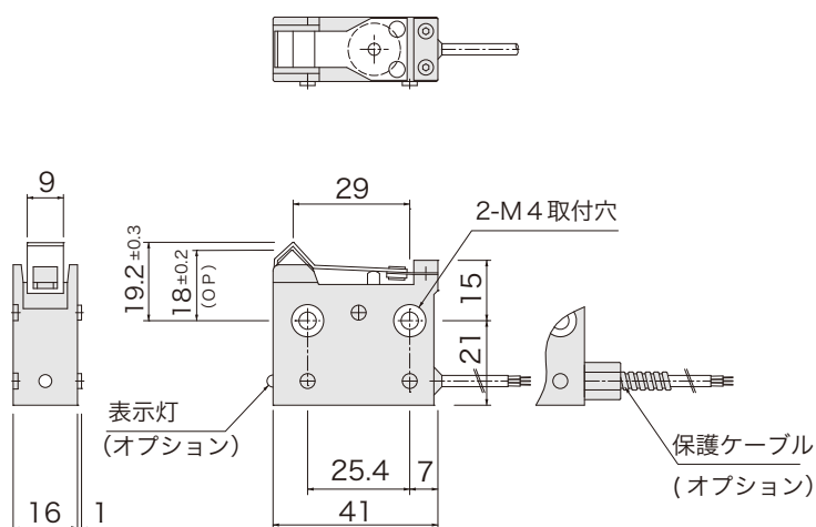
■ 外形図
