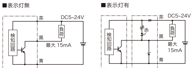
回路図
