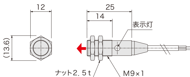
外形図
