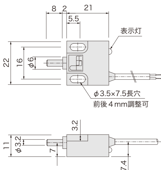
外形図
