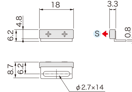
■ 外形図
