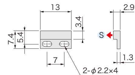
■ 外形図
