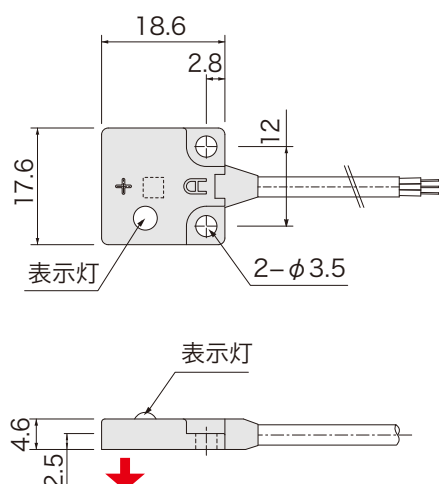
外形図
