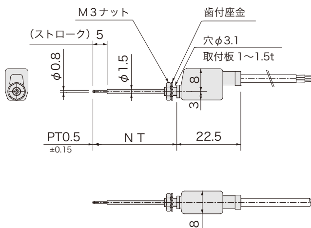
外形図
