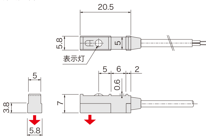
外形図
