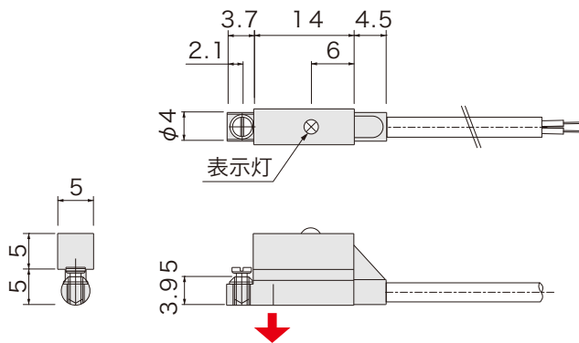
■ 外形図
