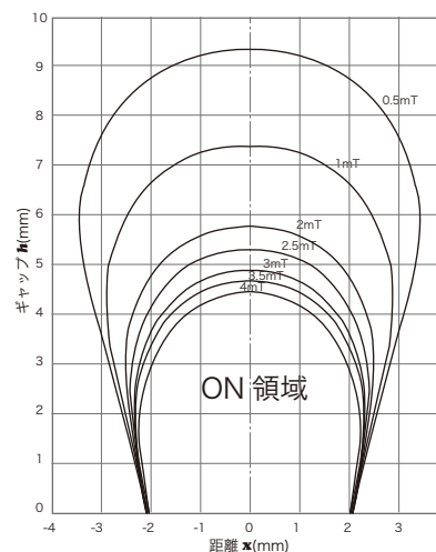
磁気特性
