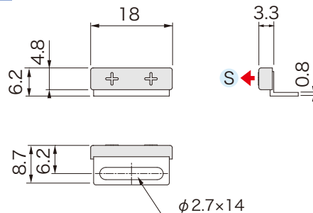
外形図
