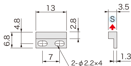
外形図
