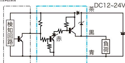
回路図
