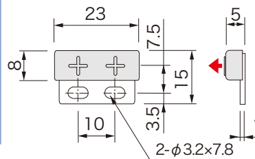
■ 外形図
