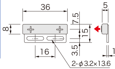
■ 外形図
