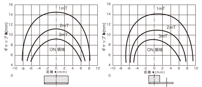
■ 磁気特性
