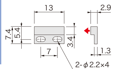
■ 外形図
