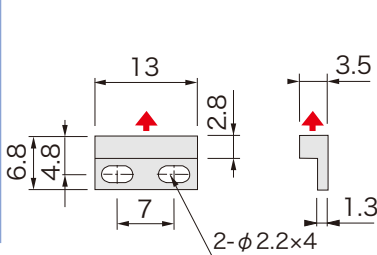
■外形図
