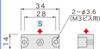
■ 外形図
