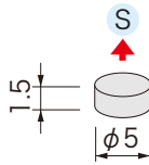
■ 外形図
