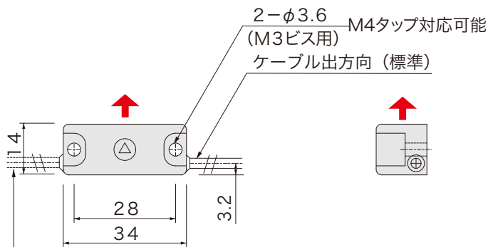
外形図
