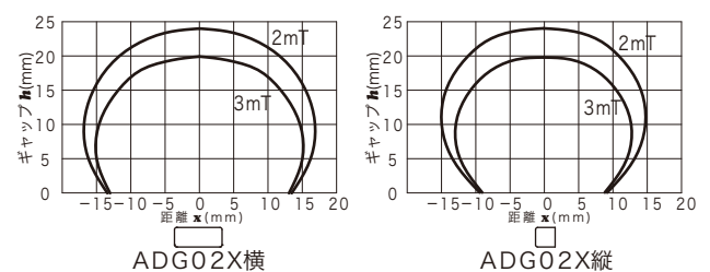
磁気特性
