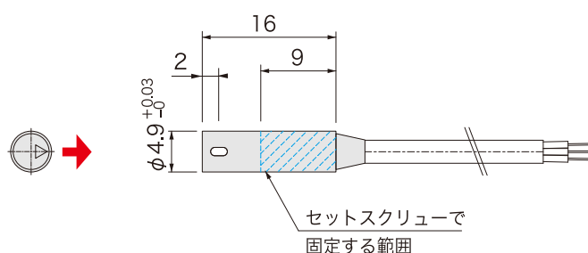
外形図
