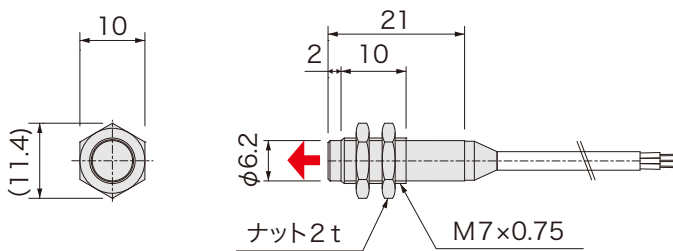
外形図
