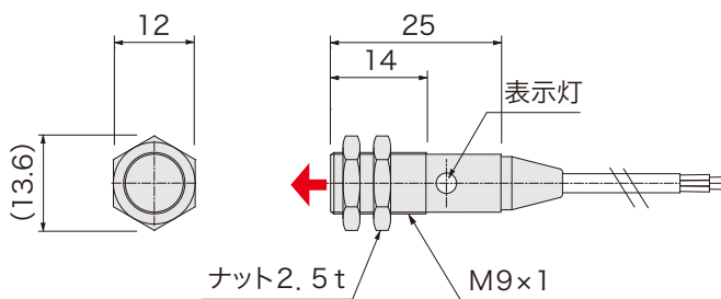
■ 外形図
