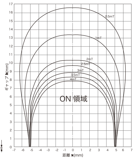
■ 磁気特性
