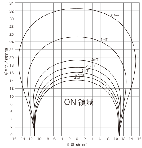
■ 磁気特性
