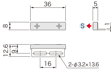
■ 外形図
