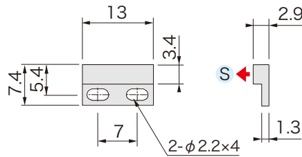
■ 外形図
