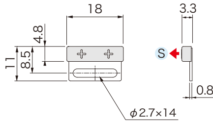
■ 外形図
