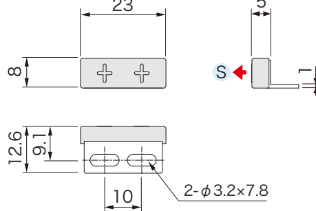
外形図
