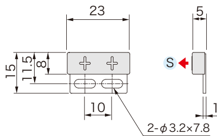
外形図
