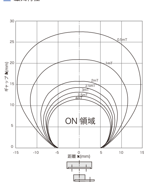
磁気特性
