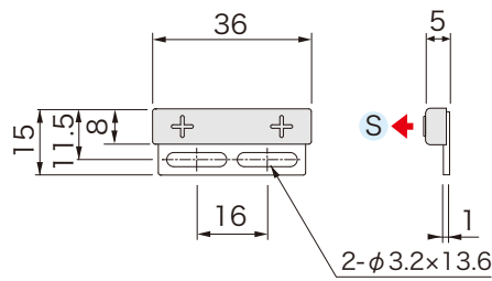
外形図
