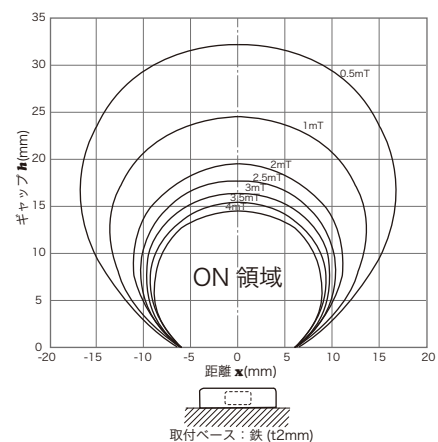
■ 磁気特性
