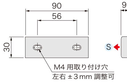
■ 外形図
