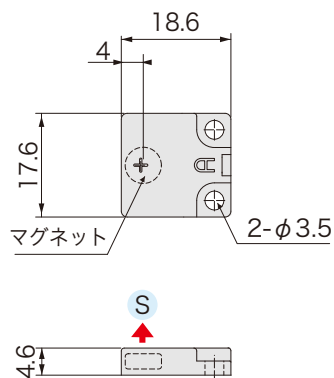
■ 外形図
