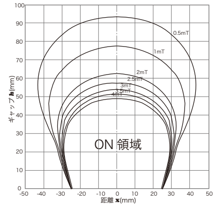
■ 磁気特性
