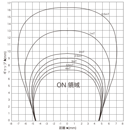
■ 磁気特性
