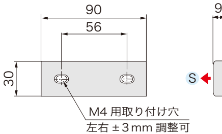
■ 外形図
