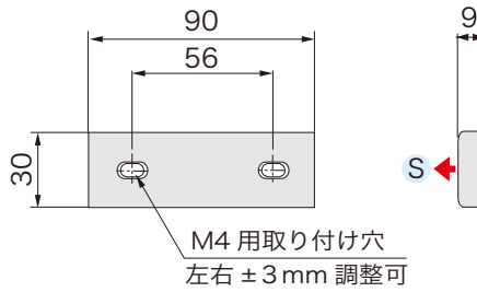
■ 外形図
