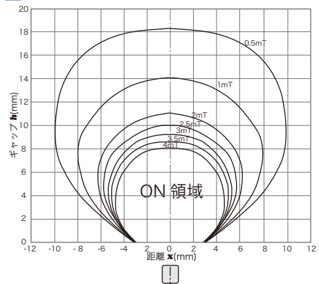
■ 磁気特性
