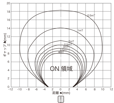
■ 磁気特性
