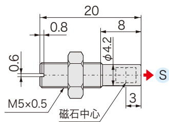
■ 外形図
