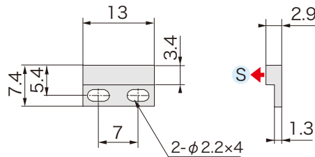
■ 外形図
