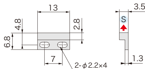
■ 外形図
